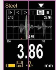
A-Scan
